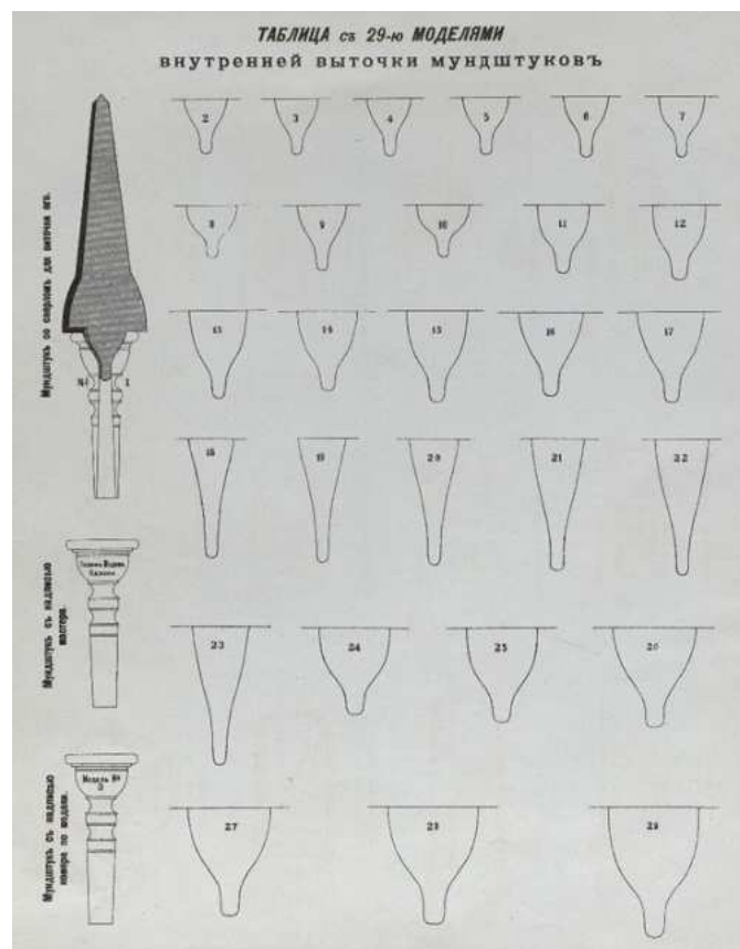
Obr. 6 | Nákresy profilových průřezů nátrubků z Šedivovy příručky.
